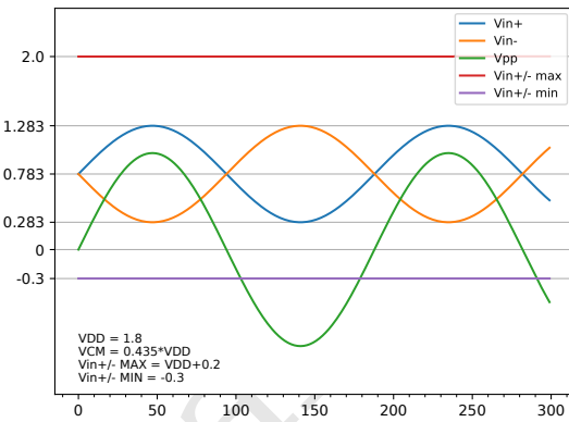
图 6: 输入信号满量程示意图
