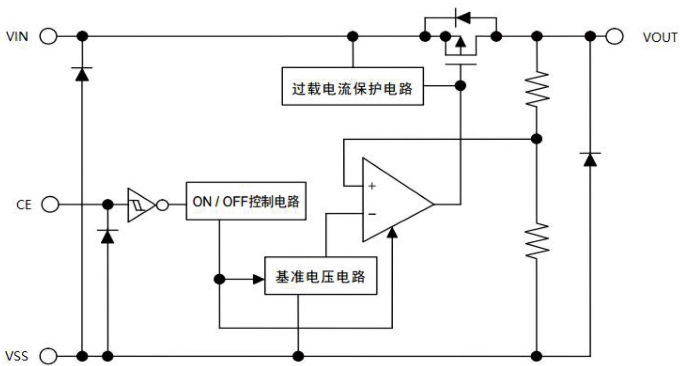
电路方框图
