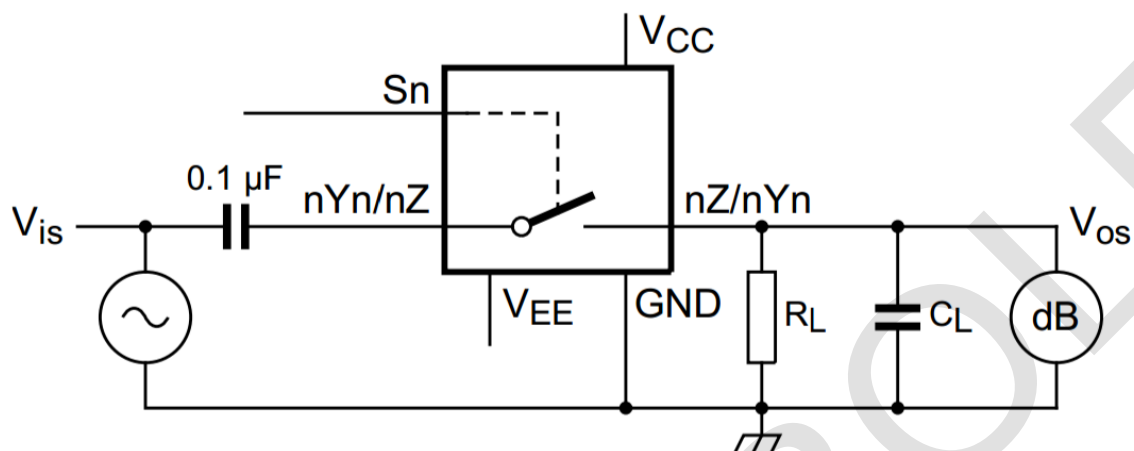
a. Test circuit
