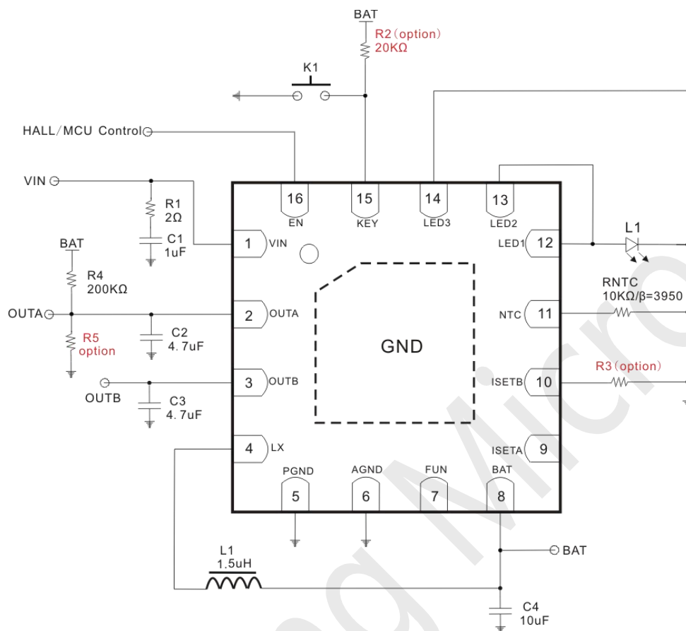
Fig8. 1 灯模式—1 (LED3 须接地)
