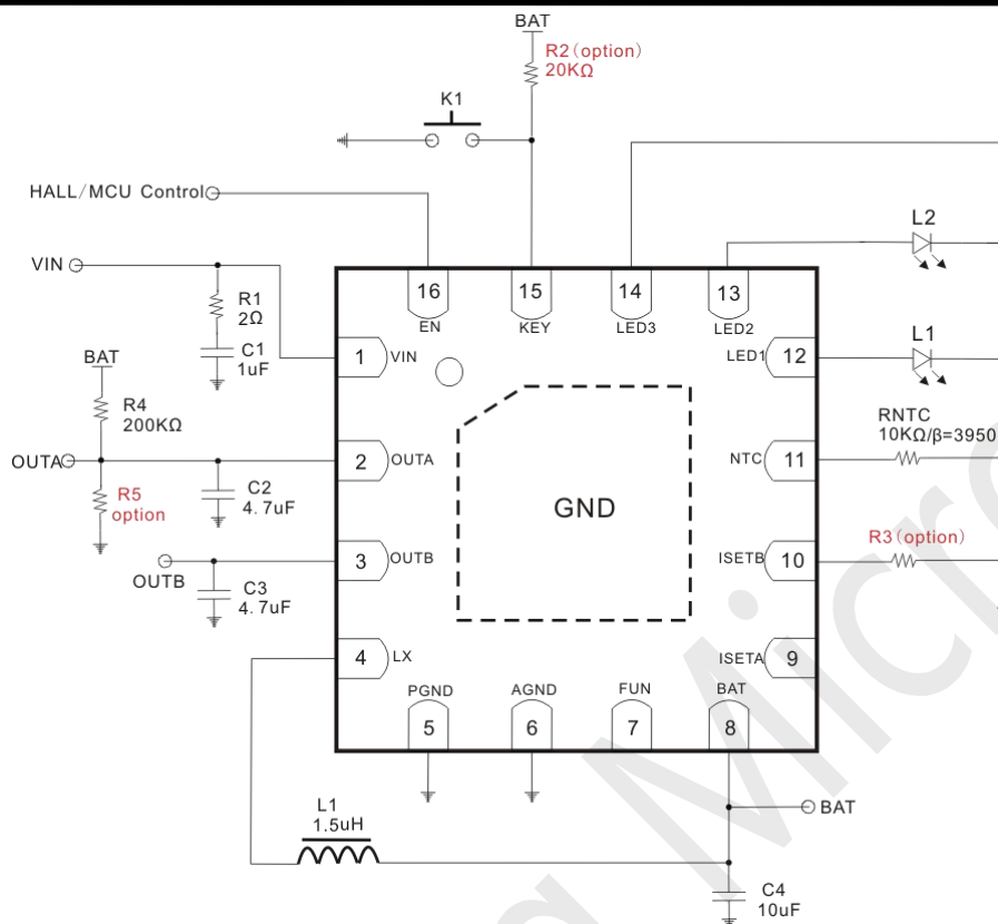
Fig7. 2 灯模式 (LED3 须接地)
