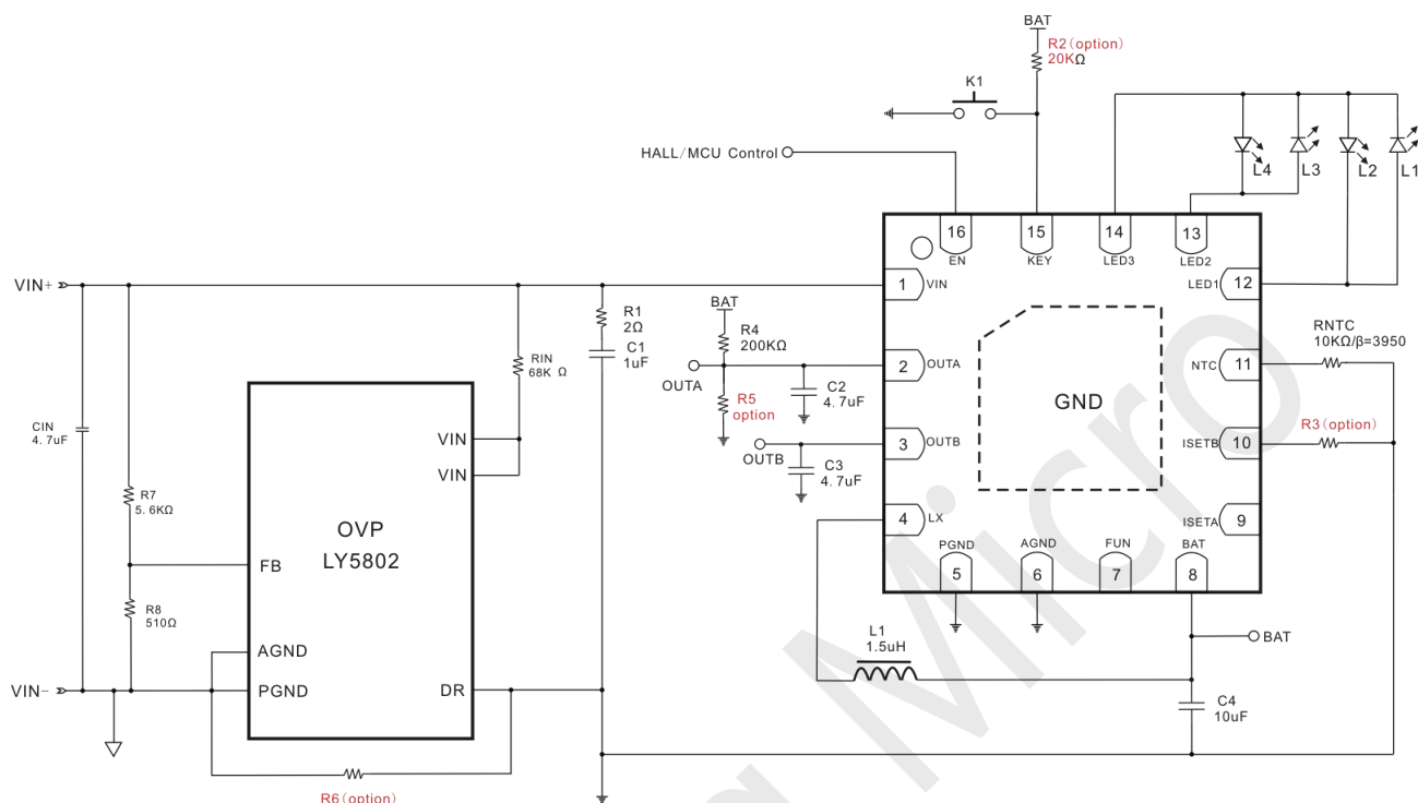
Fig2.带 OVP 应用电路
