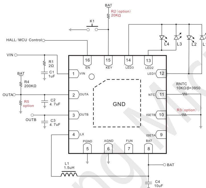
Fig5. 4 灯模式
