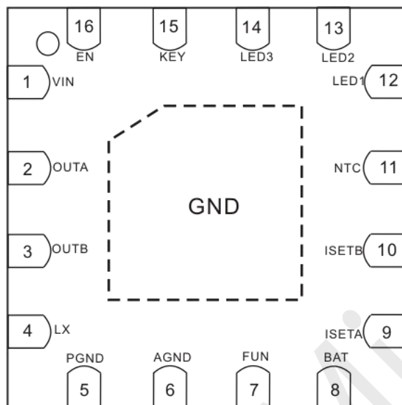
Fig4.管脚示意图
