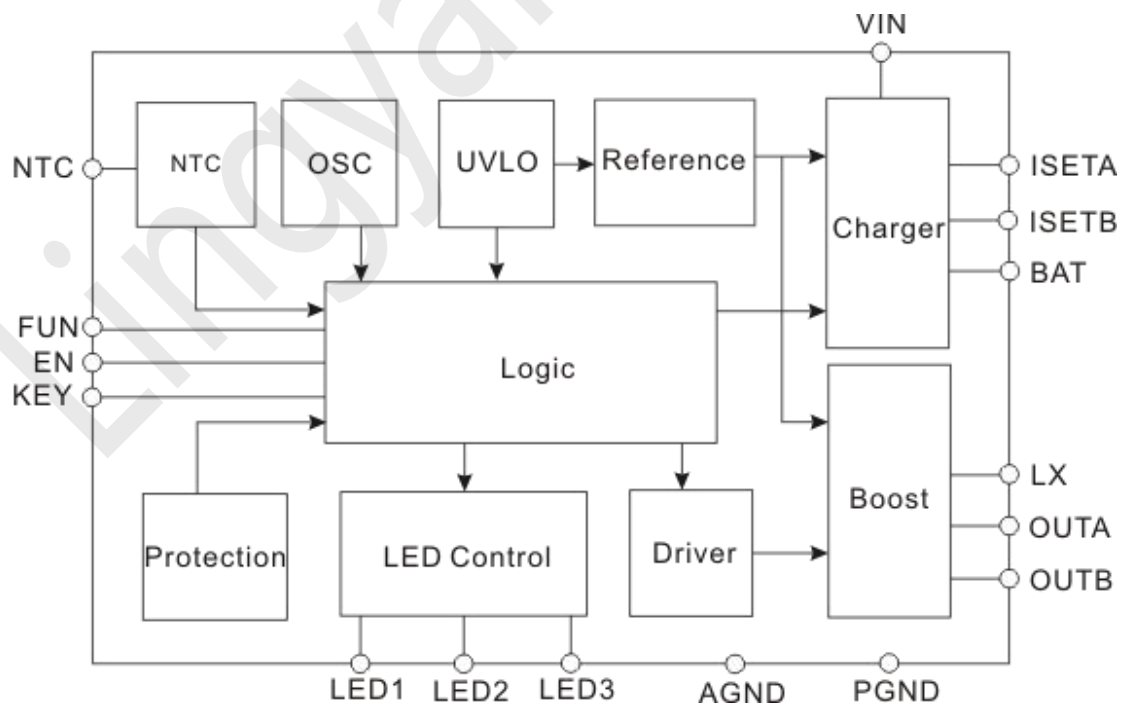
Fig3.功能框图
