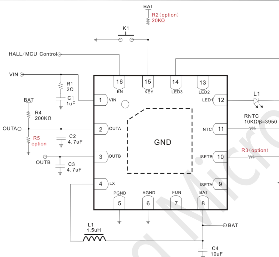
Fig9. 1 灯模式—2 (LED3 须接地)
