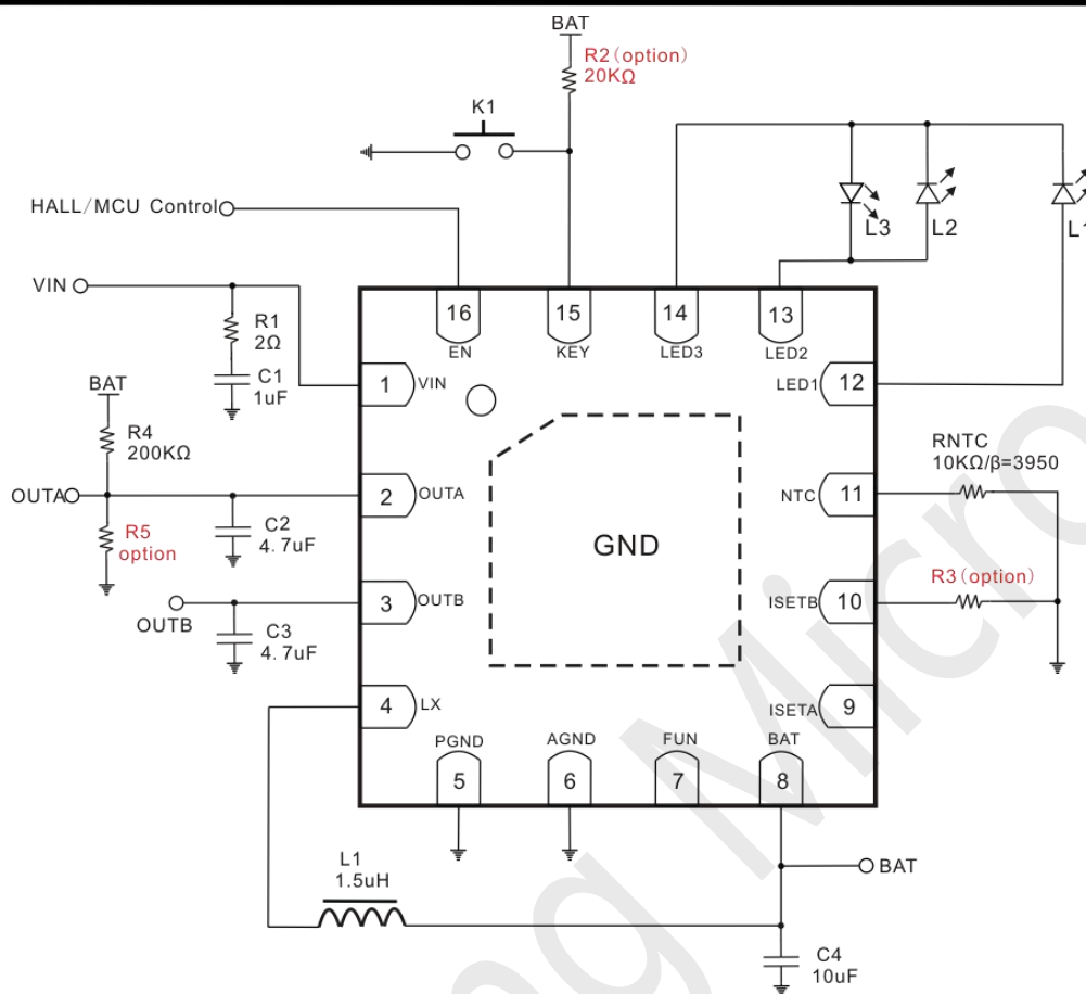
Fig6. 3 灯模式
