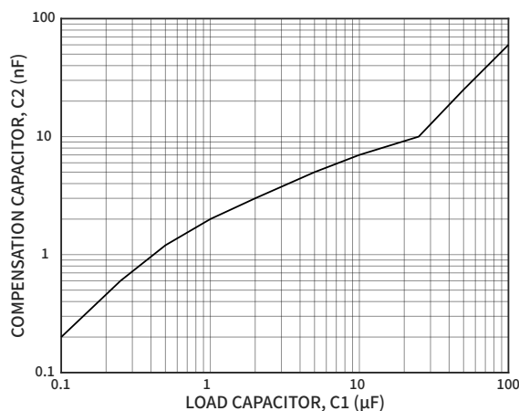
图 11 负载和补偿电容取值
