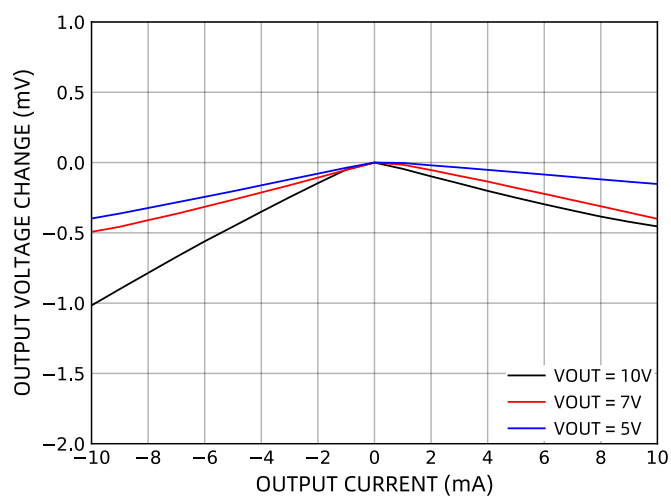
图 6 负载调整率
