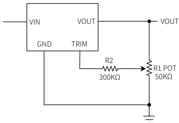
图 9 输出微调功能
