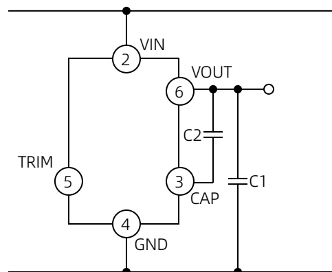
图 10 补偿电容
