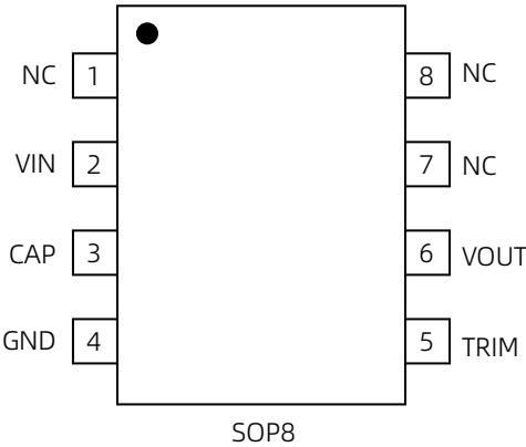
图 1 管脚示意图
