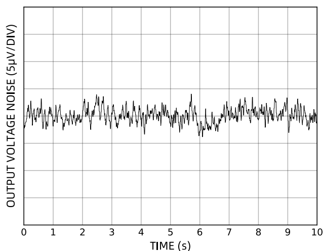
图 3 输出噪声 (7V, 0.1Hz~10Hz)
