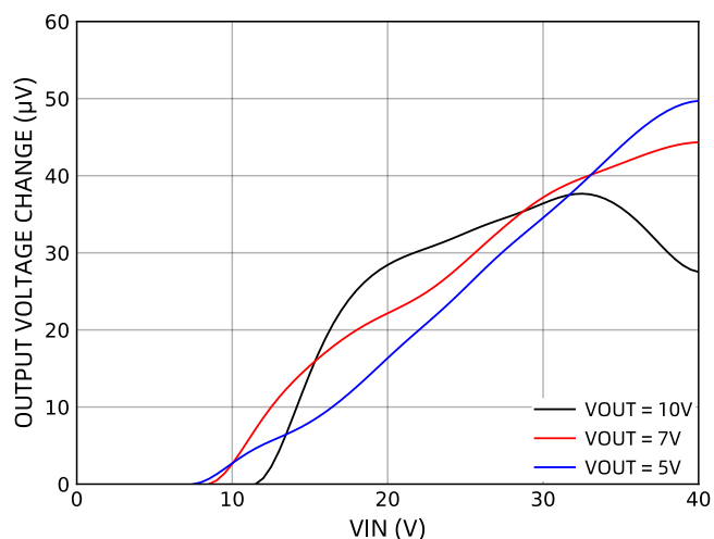
图 7 线性调整率
