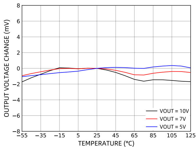
图 5 输出电压温漂
