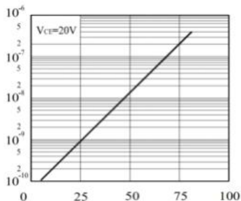
集电极暗电流与环境温度的关系
