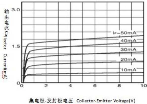
输出特性
