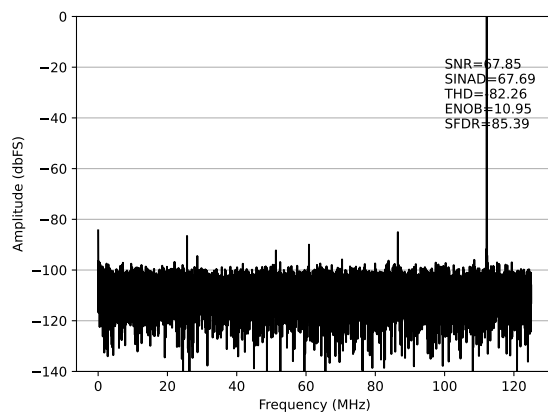
(d) 输入信号频率 = 112MHz
