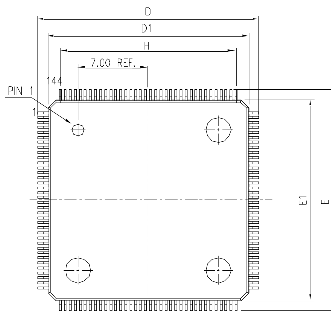
图 20 LQFP144 封装图
