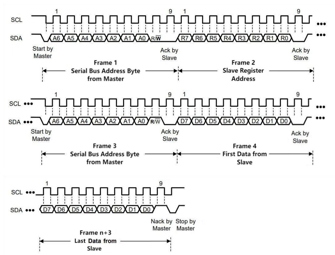
图 6.5.2-2 I2C 连续读取时序
