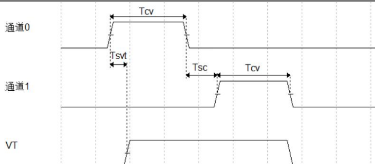
图 6.3.2-2 双通道单次转换模式工作时序图
