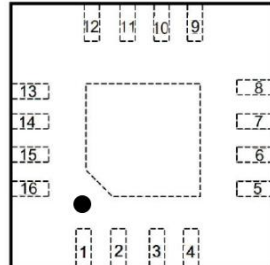
正面透视图
