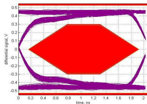
图 16. Downstream Port 3
