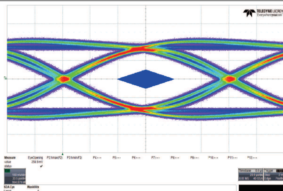
图 14. Downstream Port 1
