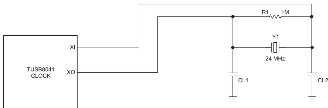
图 3. TUSB8041 Clock
