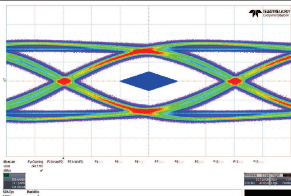
图 15. Downstream Port 2
