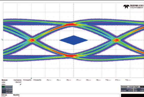
图 13. Upstream Port
