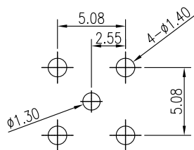
参考孔位图
