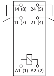
DPST (2NO)
