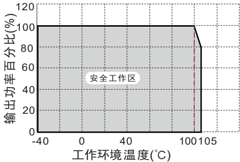
3. 3V输入 温度降额曲线图
