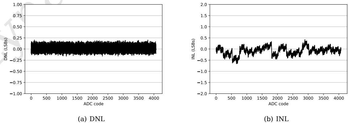
图 3: 线性特性
