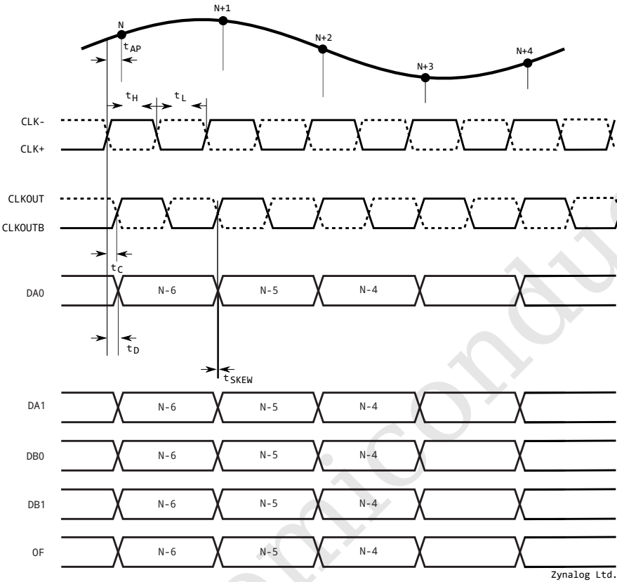
图 5: 数据输出
