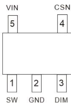
D3815C-TD(SOT23-5)
