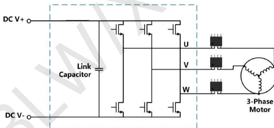
3 相电机控制应用电路
