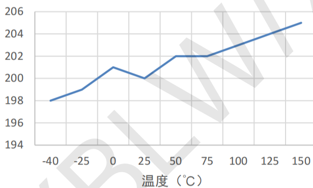
10A 灵敏度随温度变化
