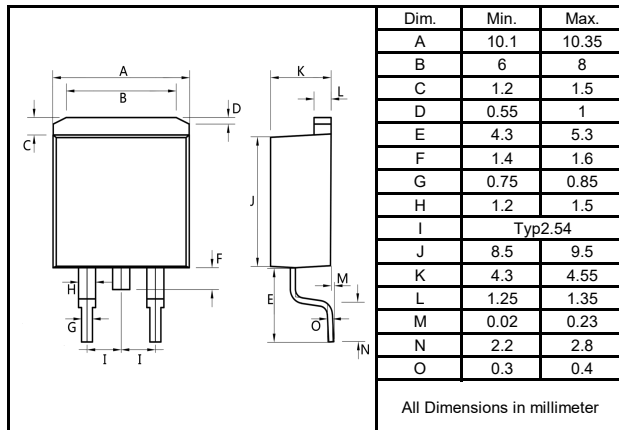
T0-263
