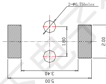
PCB. 焊接图
