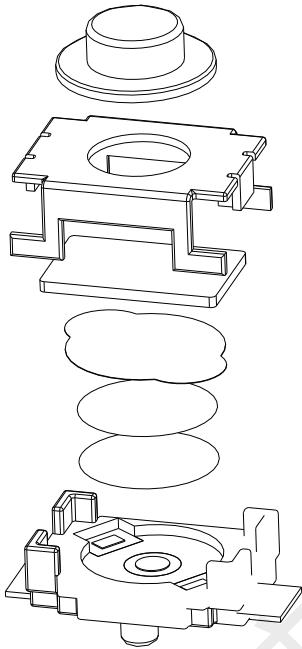
3D轴测图
