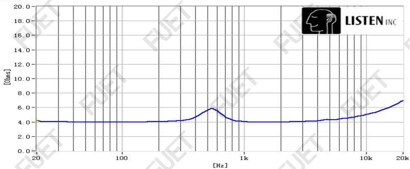
阻抗曲线
