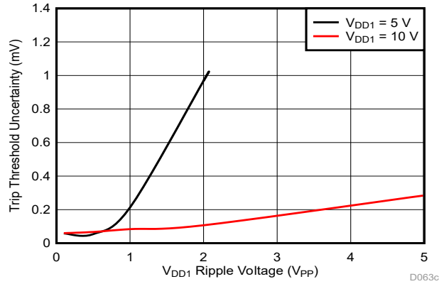
图 7-7. 跳变阈值对 VDD1 纹波电压的灵敏度 ( Cmp2 , f_{\text{RIPPLE}} = 10\text{kHz} )
