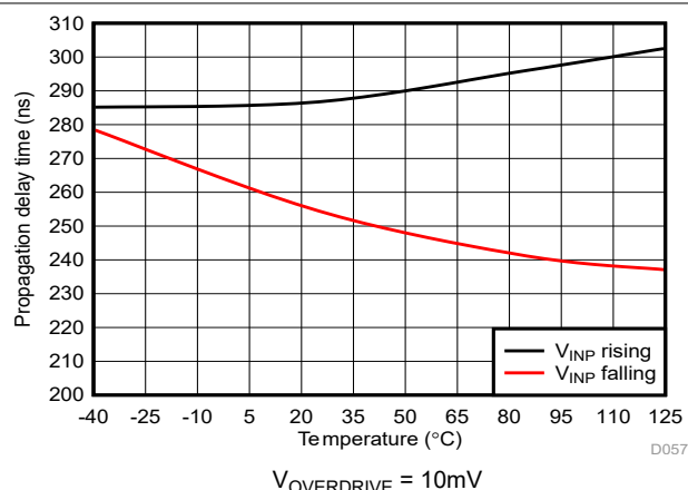
图 5-53. Cmp0 传播延迟与温度间的关系
