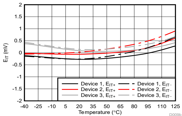
图 5-7. Cmp2 跳变阈值与温度间的关系
