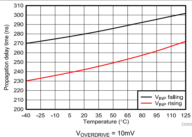
图 5-51. Cmp3 传播延迟与温度间的关系
