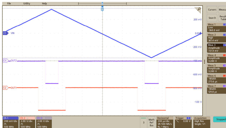
图 7-4. AMC23C14 对三角输入波形的输出响应
