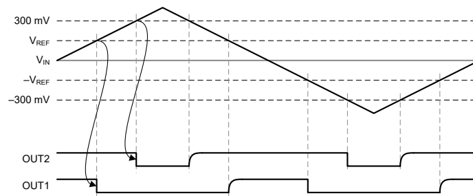
图 5-2. 功能时序图
