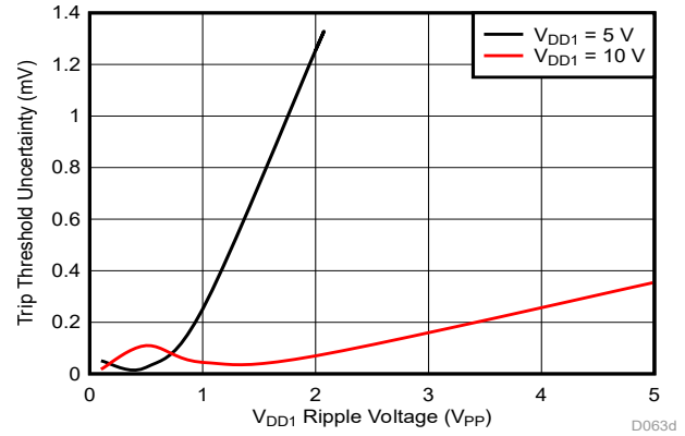
图 7-8. 跳变阈值对 VDD1 纹波电压的灵敏度 ( Cmp3 , f_{\text{RIPPLE}} = 10\text{kHz} )
