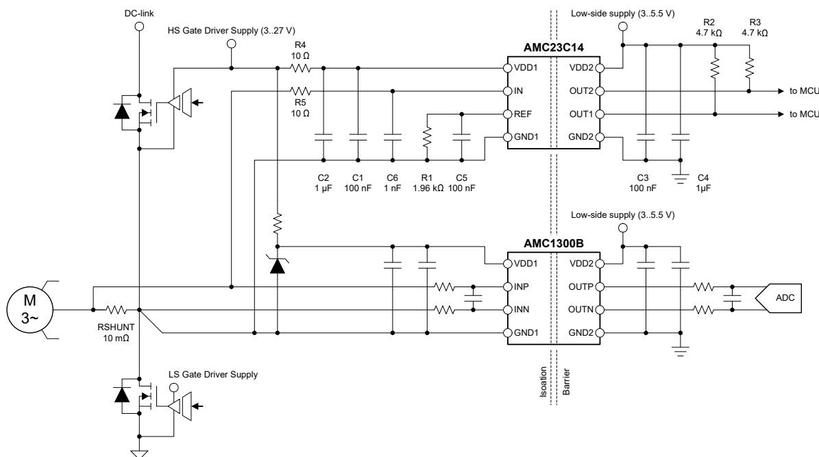
图 7-1. 使用 AMC23C14 进行过流和短路检测
