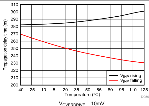
图 5-49. Cmp2 传播延迟与温度间的关系
