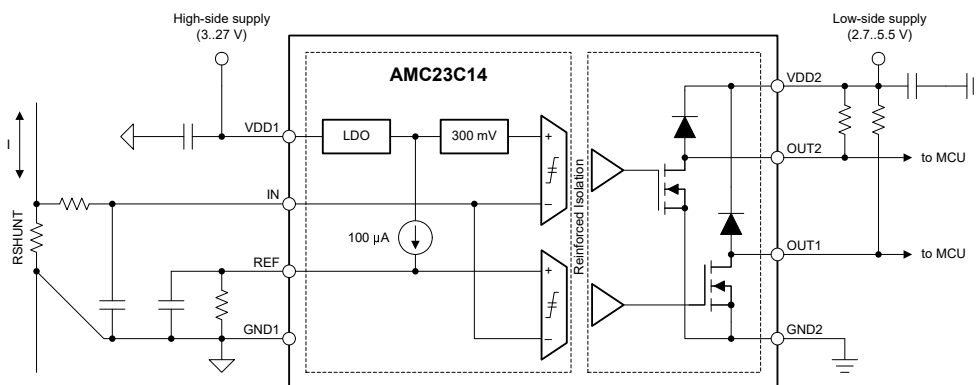
典型应用
