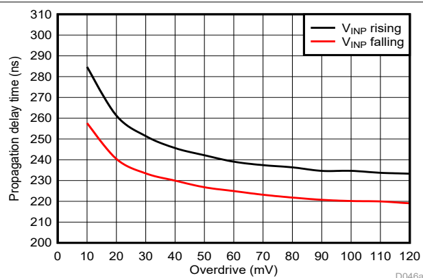
图 5-50. Cmp3 传播延迟与过驱间的关系
