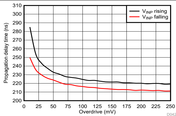
图 5-48. Cmp2 传播延迟与过驱间的关系
