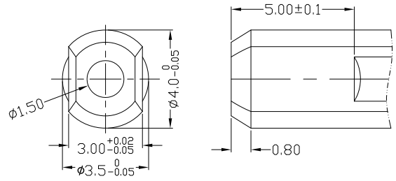
轴心部尺寸详图 2:1
