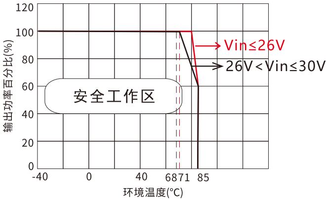
6.5V/9V/12V/15V 正输出 温度降额曲线图
