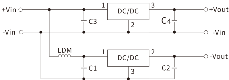
正负输出并联应用电路
