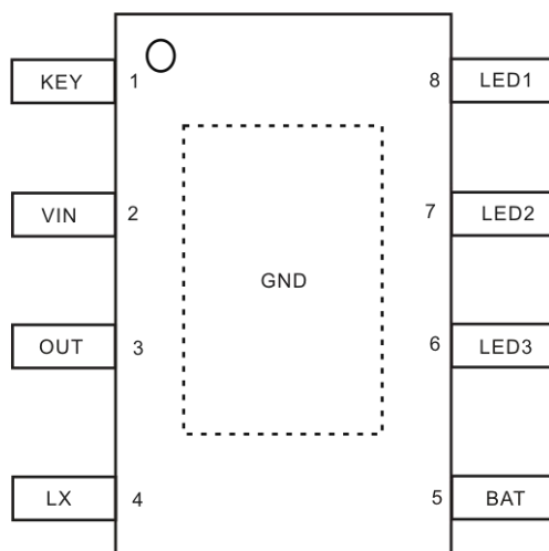
Fig4.管脚示意图
