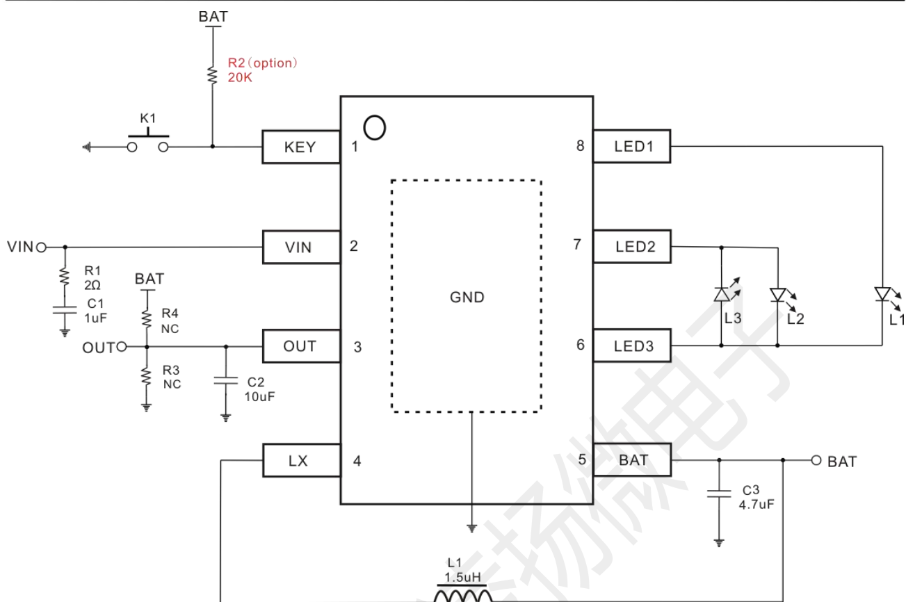
Fig6. 3 灯模式
