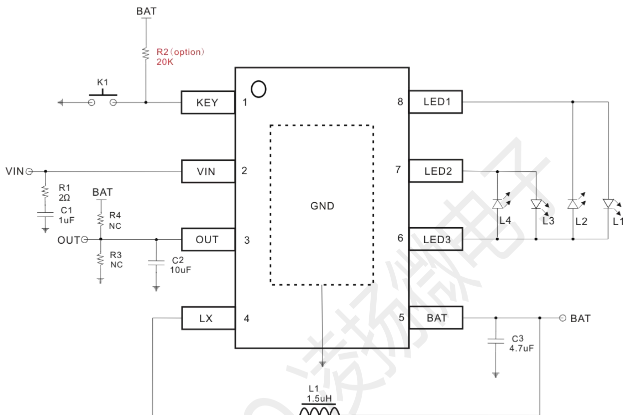
Fig5. 4 灯模式
