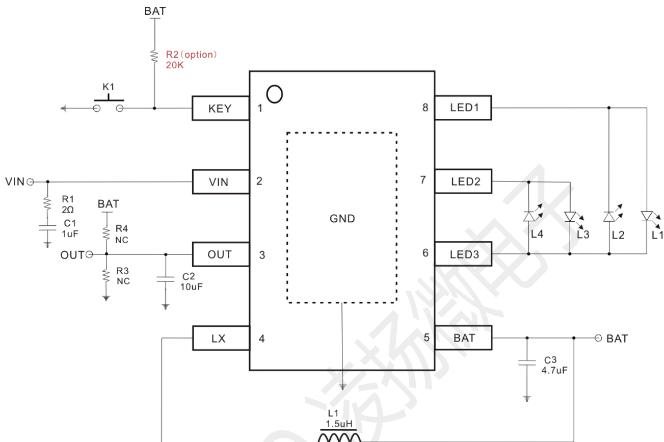
Fig1.LY6394 典型应用电路
