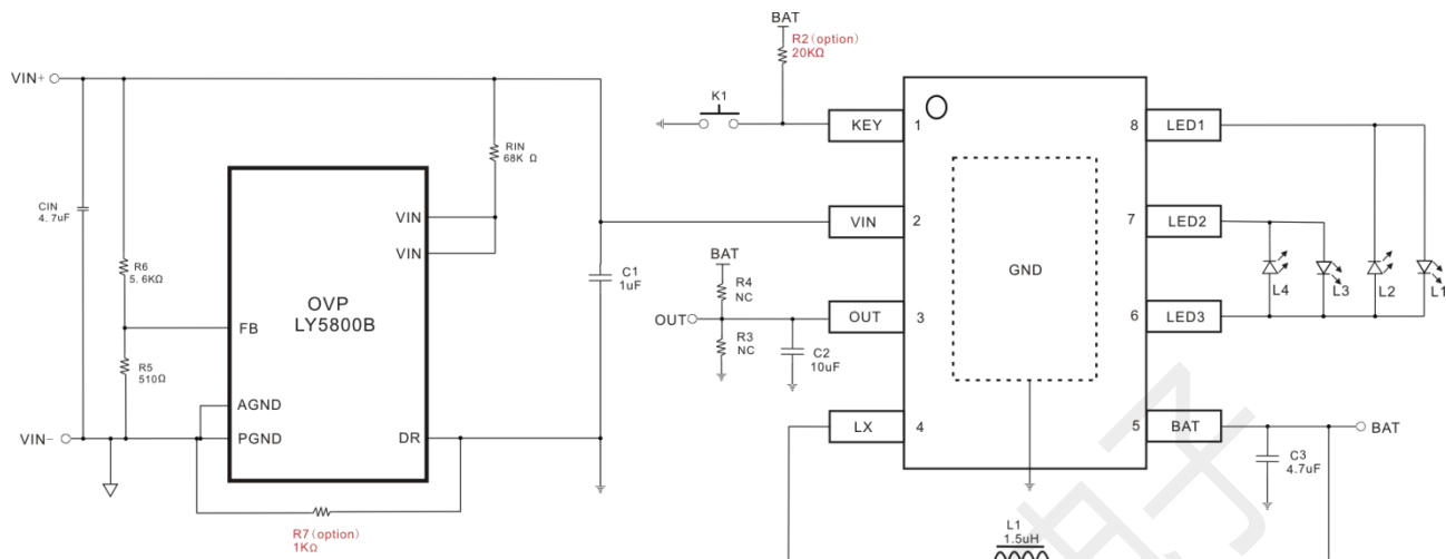
Fig2.帶 OVP 应用电路
