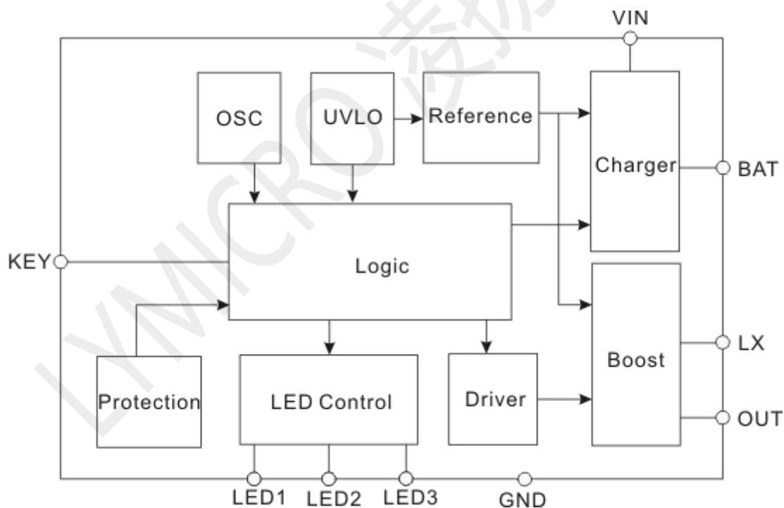
Fig3.功能框图
