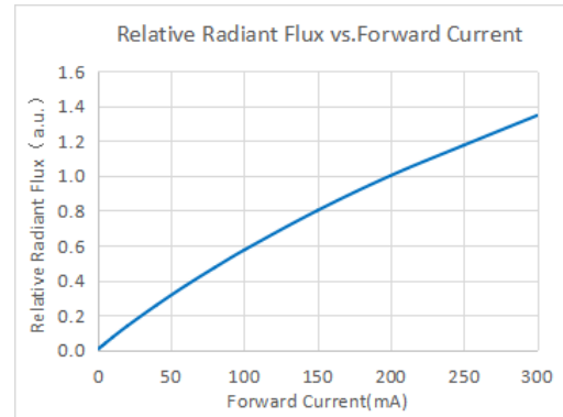
2) 正向电流与相对辐射通量特性曲线
