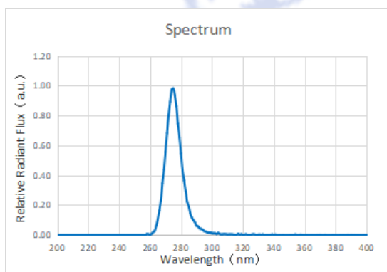
5) 光谱分布特性曲线
