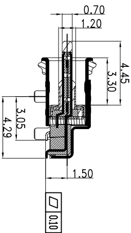
SECTION A-A(SCALE 1:1)
