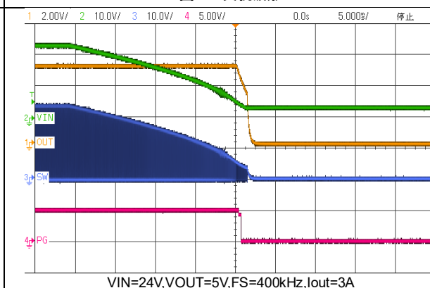
图 19. 关机波形
