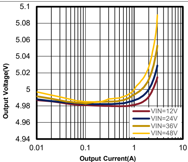
图 10. F_S=1MHz VOUT 特性
