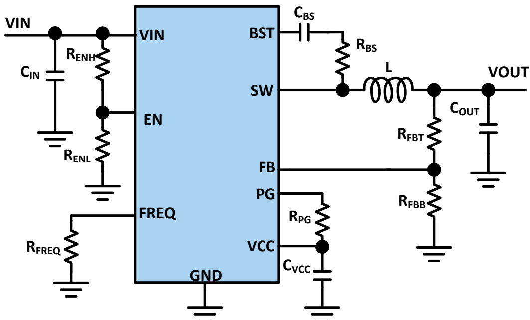
图2 DC-DC 降压模式典型应用拓扑
