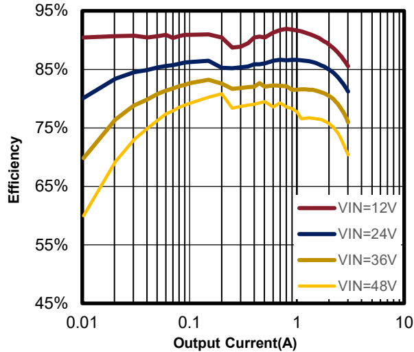
图 7. F_S=1MHz 效率
