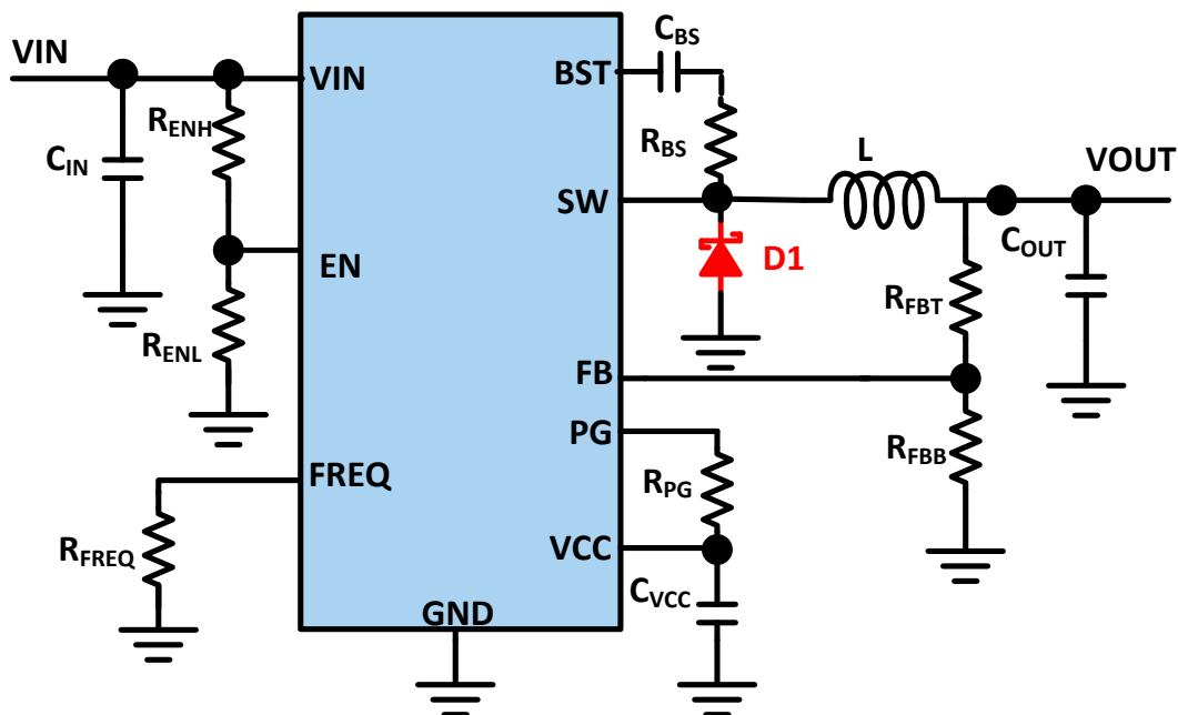
图4 DC-DC 输入高压大电流应用拓扑
