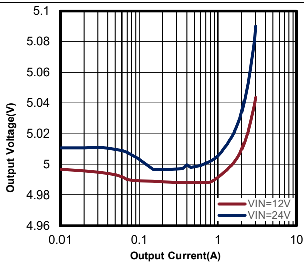
图 11. F_S=2MHz VOUT 特性
