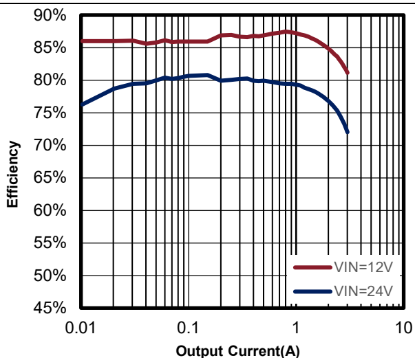
图 8. F_S=2MHz 效率
