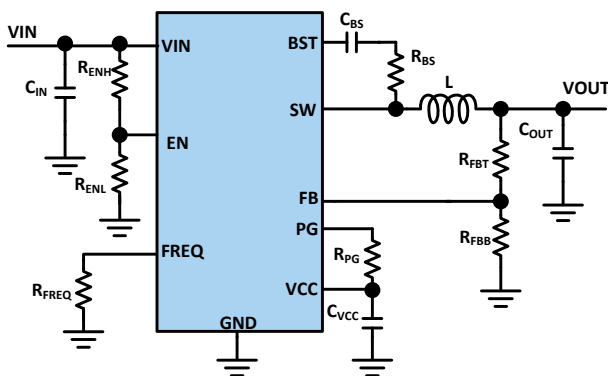
图 1 典型应用拓扑
