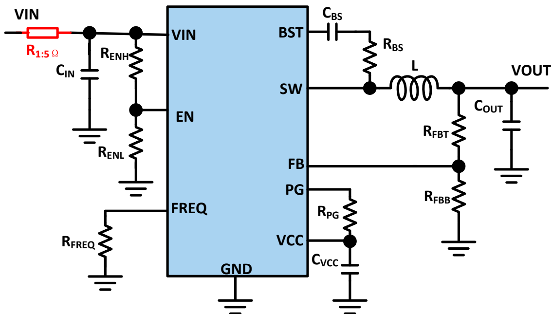
图3 DC-DC 降压模式热插拔应用拓扑
