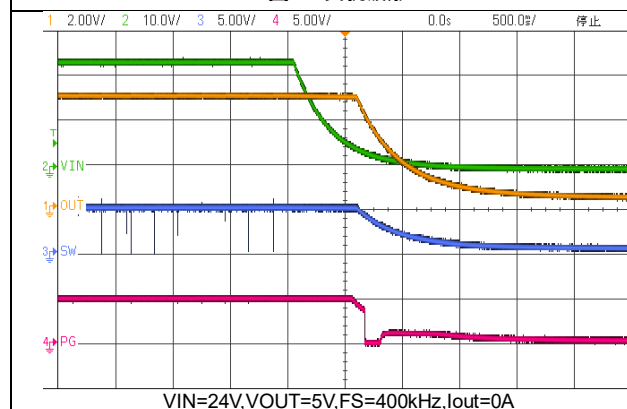
图 18. 关机波形
