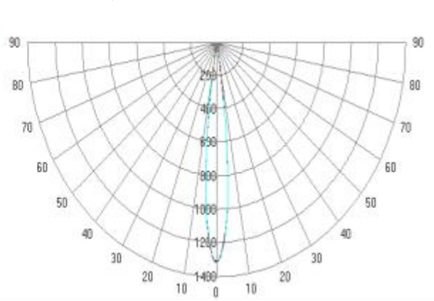
配光曲线-极坐标
