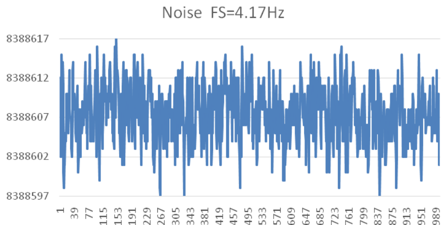
MS5199T 噪声 (AVDD=4V, 基准电压 = 2.048, 增益= 64, 更新速率 = 4.17 Hz)
