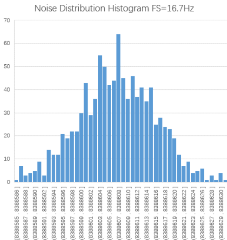
MS5199T 噪声分布柱状图 (AVDD=4V, 基准电压 = 2.048, 增益= 64, 更新速率= 16.7 Hz)
