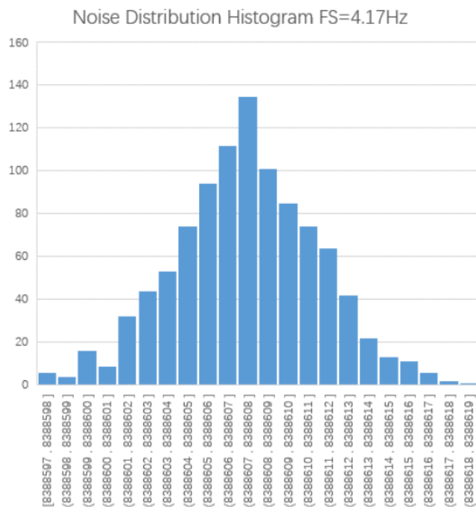
MS5199T 噪声分布柱状图 (AVDD=4V, 基准电压= 2.048, 增益= 64, 更新速率= 4.17 Hz)
