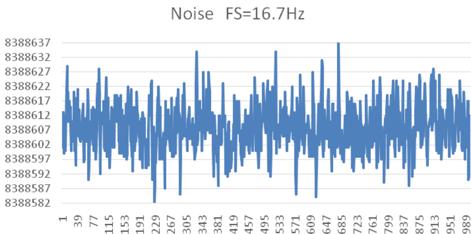
MS5199T 噪声 (AVDD=4V, 基准电压 = 2.048, 增益= 64, 更新速率 = 16.7 Hz)
