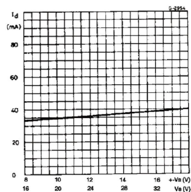
图 9 静态电流 VS 电频率 响应源电压
