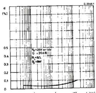
图 7 失真 VS 频率
