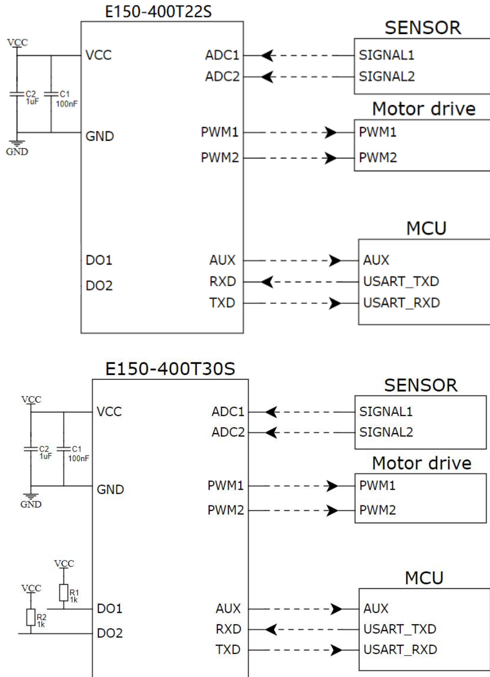
连接 MCU 示意图
