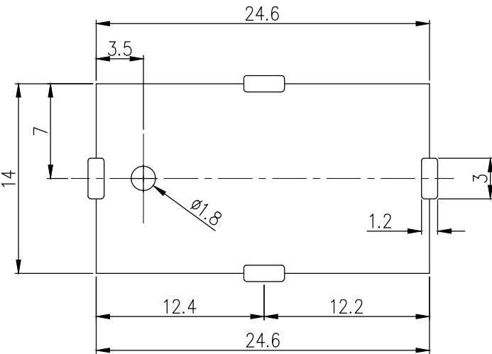
P. C. B 参考图
