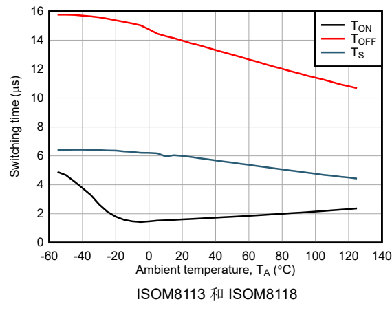
图 6-29. 开关时间与环境温度间的关系
