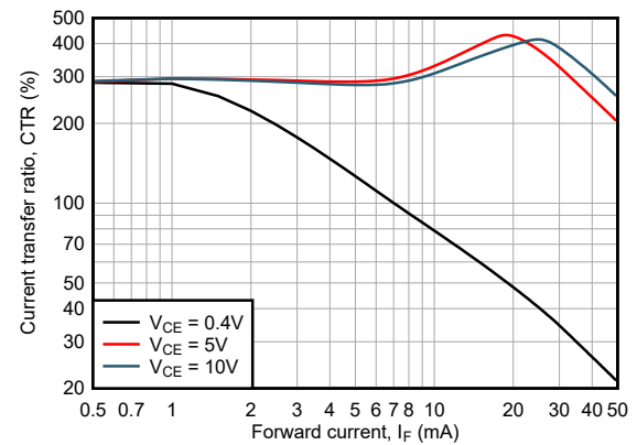
ISOM8112 和 ISOM8117 T_A = 25^\circ C
