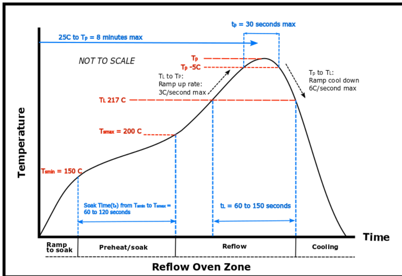
图 9-8. TI 对 J-STD-020 分类曲线的表示 ( 非按比例绘制 )
