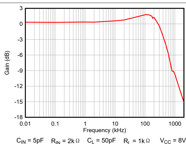
图 9-3. R_L = 1k\Omega 时的带宽
