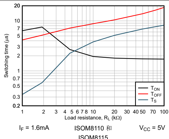
图 6-22. 开关时间与负载电阻间的关系
