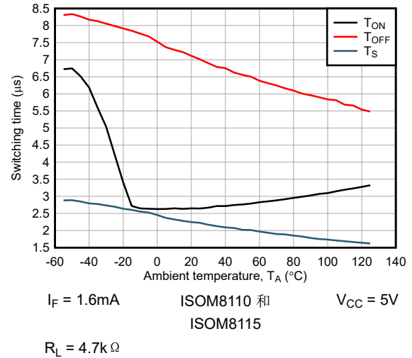
图 6-26. 开关时间与环境温度间的关系
