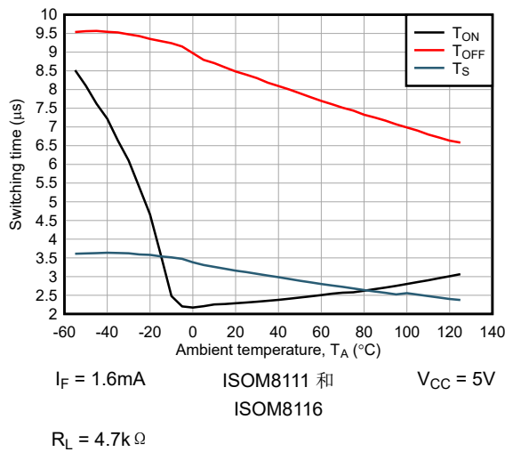
图 6-27. 开关时间与环境温度间的关系
