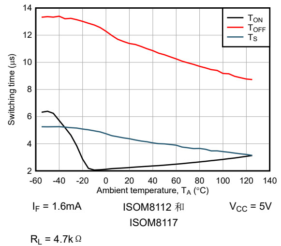
图 6-28. 开关时间与环境温度间的关系
