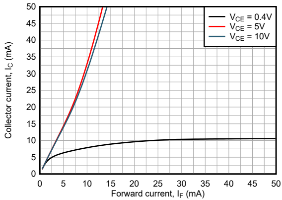
ISOM8112 和 ISOM8117 T_A = 25^\circ\text{C}
