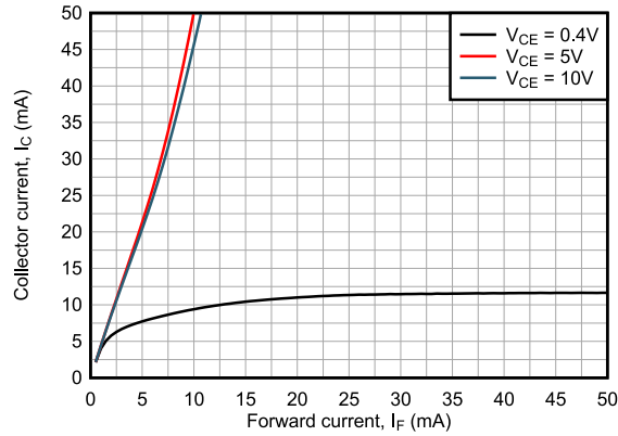
ISOM8113 和 ISOM8118 T_A = 25^\circ C
