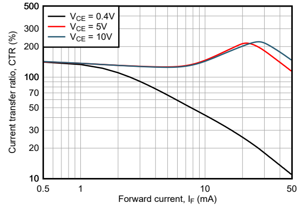
ISOM8110 和 ISOM8115 T_A = 25^\circ C
