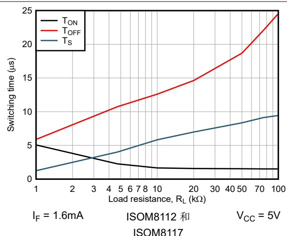
图 6-24. 开关时间与负载电阻间的关系
