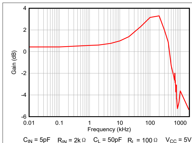
图 9-2. R_L = 100\Omega 时的带宽
