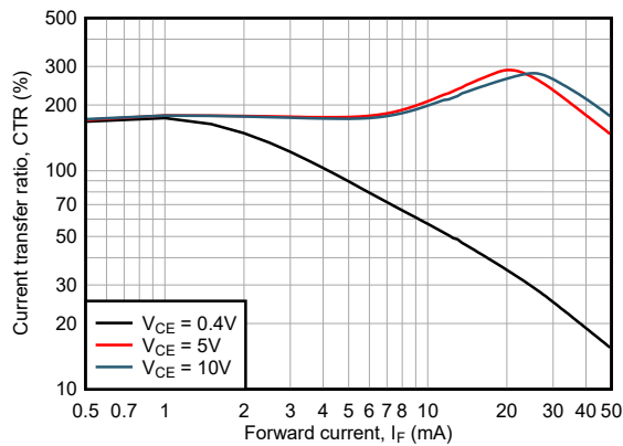
ISOM8111 和 ISOM8116 T_A = 25^\circ C
