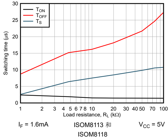
图 6-25. 开关时间与负载电阻间的关系
