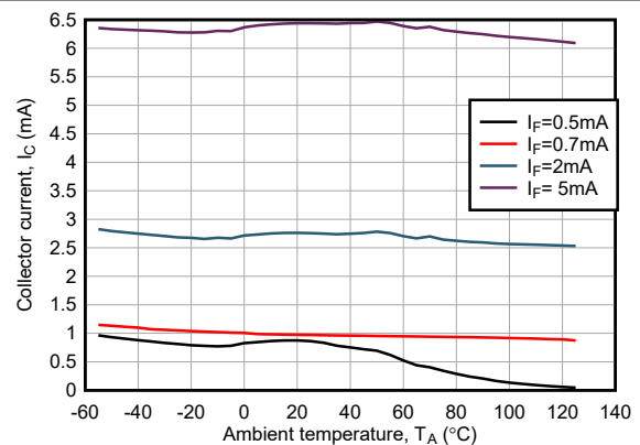
ISOM8110 和 ISOM8115 V_{CE} = 5V
