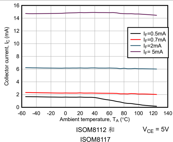
图 6-20. 集电极电流与环境温度间的关系
