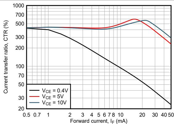
ISOM8113 和 ISOM8118 T_A = 25^\circ C
