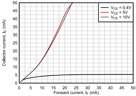
ISOM8110 和 ISOM8115 T_A = 25^\circ\text{C}
