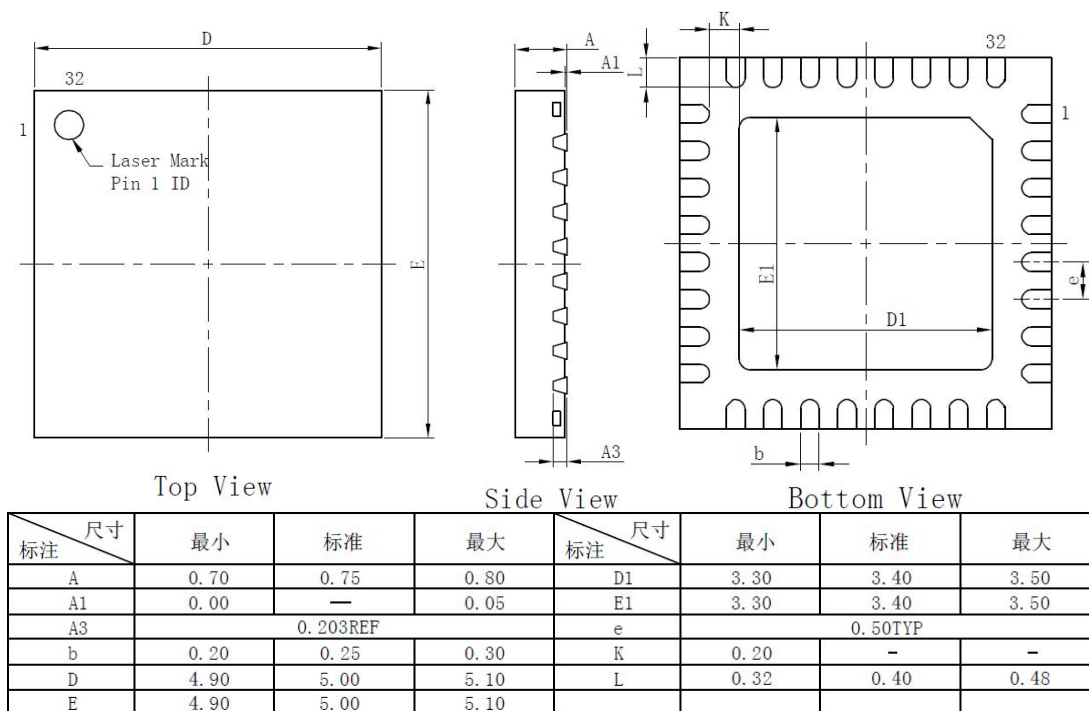
图 4 QFN32 封装信息
