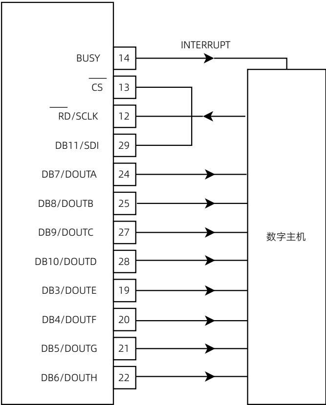
图 65 接口图-串行接口 8 条 \text{DOUTx} 线路
