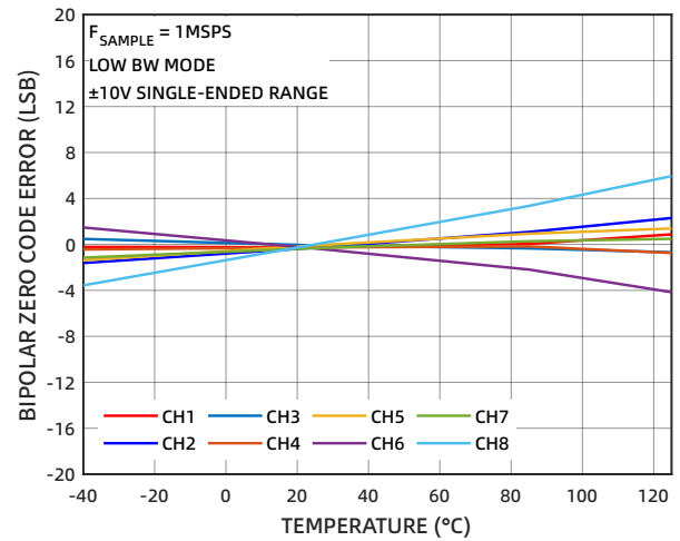
图 21 0 码误差的温度特性 (±10V 单端输入)
