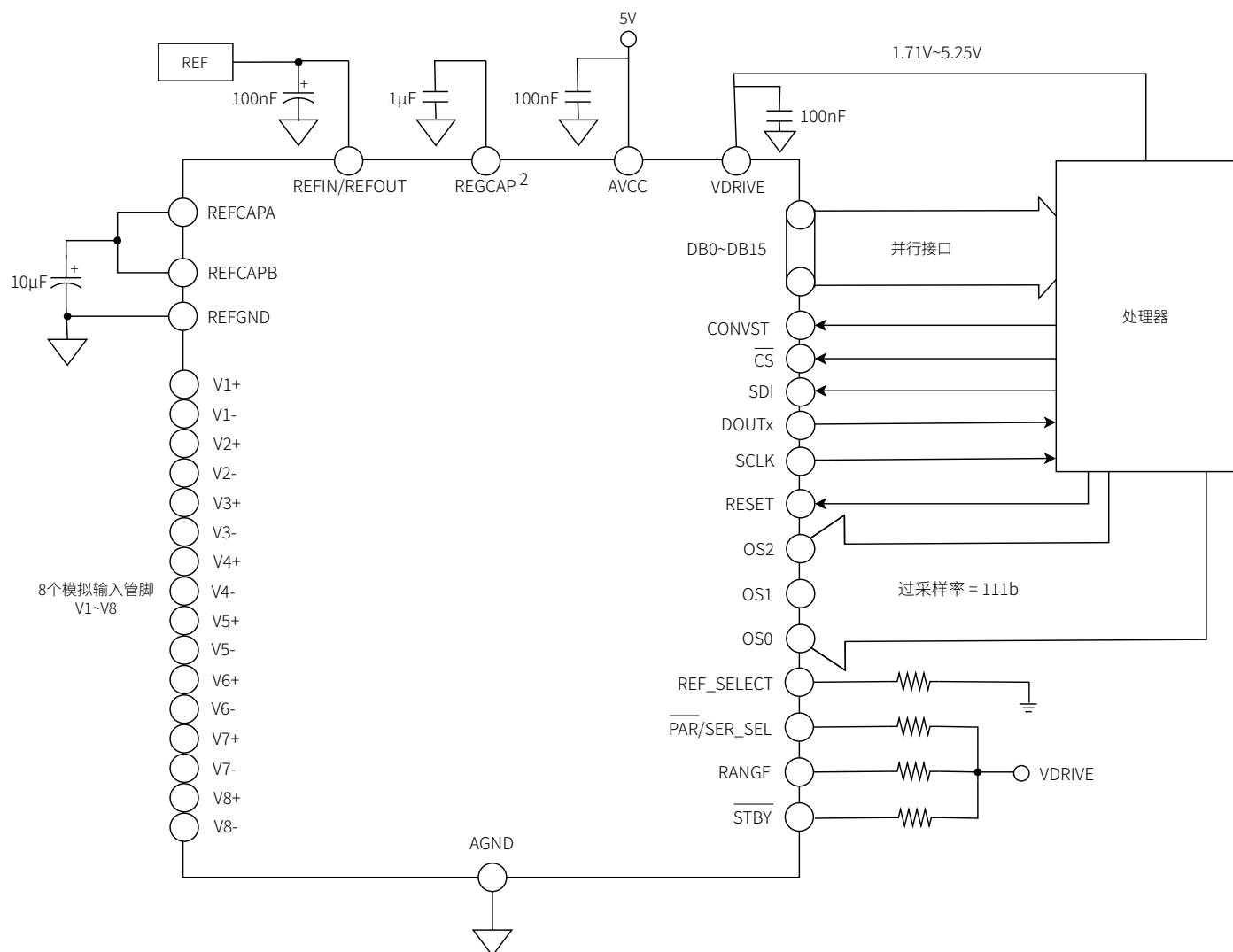
图 78 软件模式典型连接图
