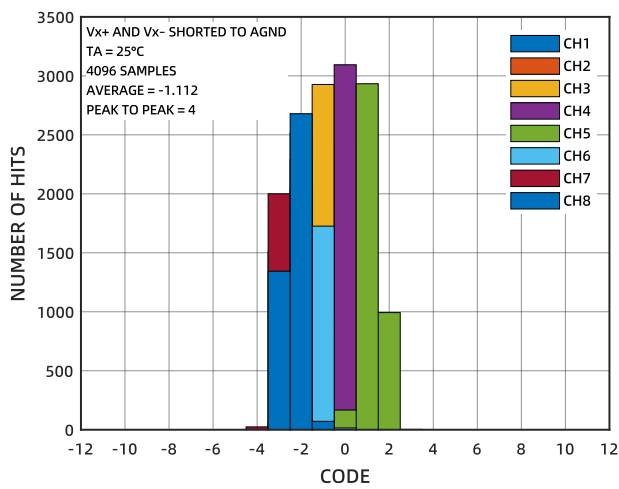
图 22 零输入直方图 (±20V 差分输入)
