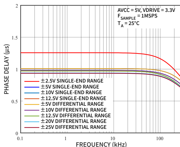
图 42 模拟抗混叠滤波器相频特性，高带宽模式
