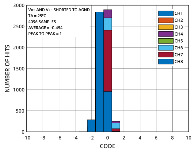
图 23 零输入直方图 (±10V 单端输入)
