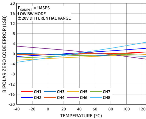
图 20 0 码误差的温度特性 (±20V 差分输入)
