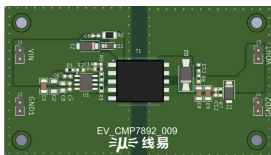
图 3.2 PCB 示意图 (尺寸: 80 x 45mm)
