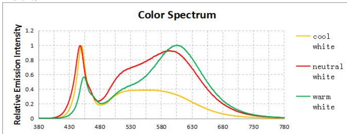
光谱图, T_a=25^\circ\text{C}
