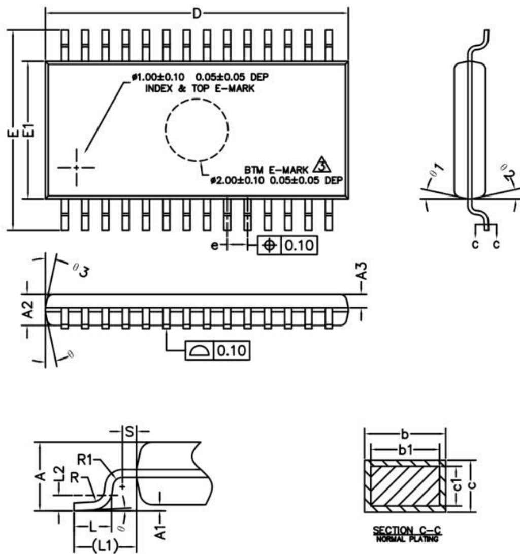
TSSOP28 9.6*4.3, 封装尺寸 POD 图,
