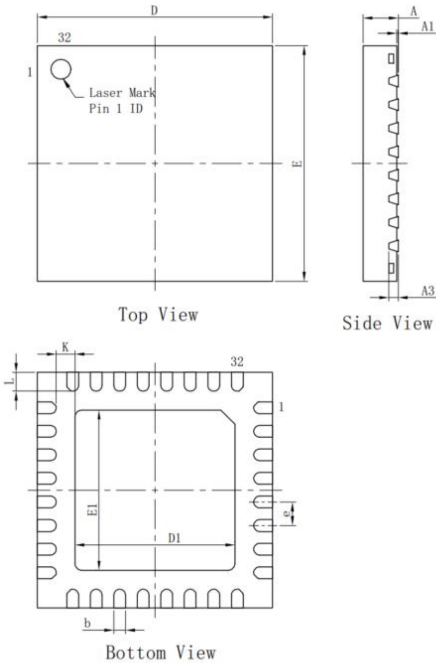
QFN32 5*5, 封装尺寸 POD 图
