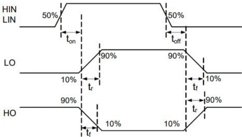
图 26 开关时序
