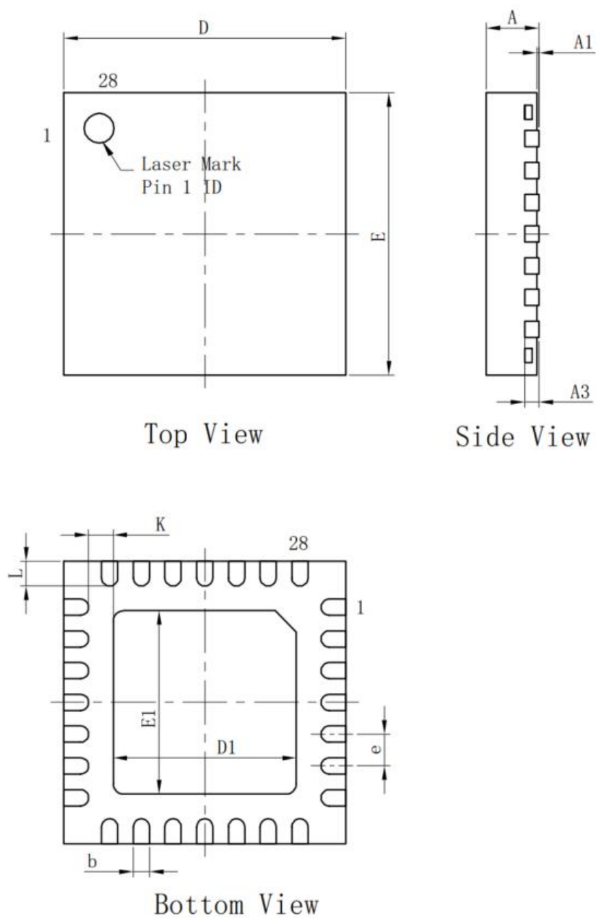
QFN28 4*4, 封装尺寸 POD 图,
