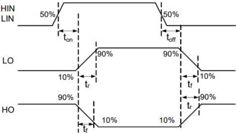
图 22 开关时序
