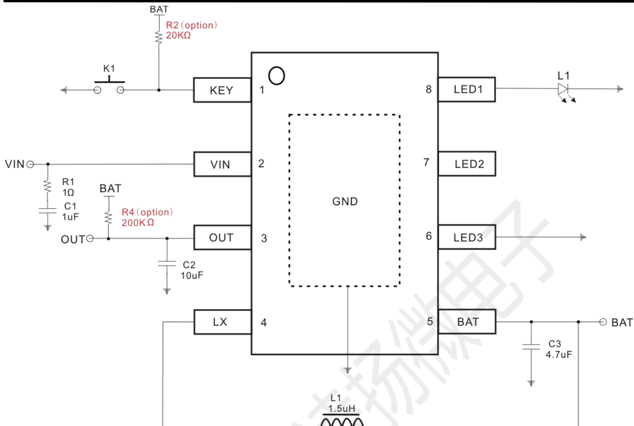
1 灯模式—2 (LED3 须接地)
