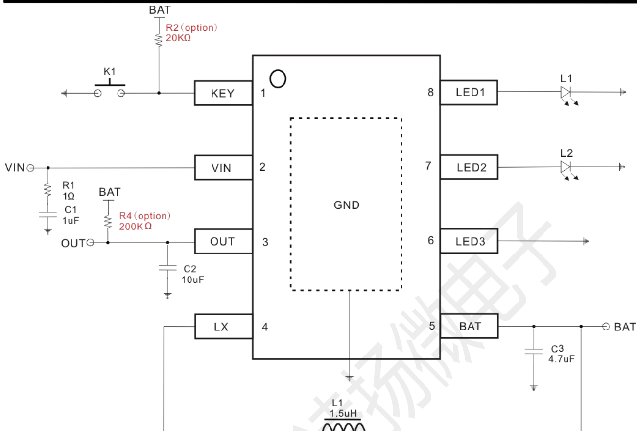
2 灯模式 (LED3 须接地)
