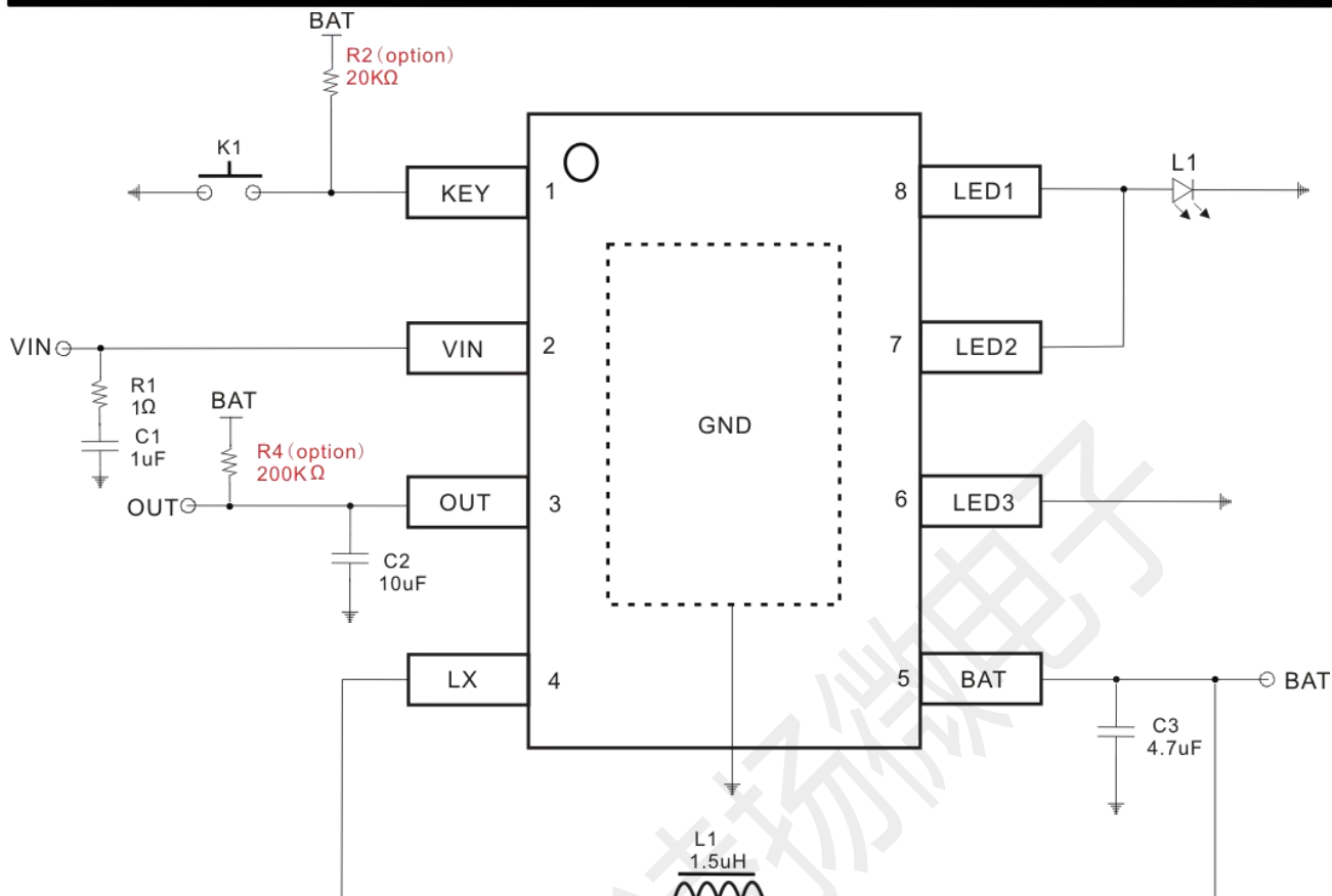
1 灯模式—1 (LED1 和 LED2 接一起, LED3 须接地)
