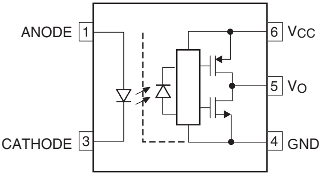
TLP155 功能框图 (1)
