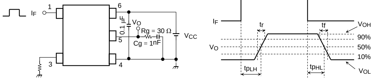
图 1: t_{PLH} , t_{PHL} , t_r , t_f , |t_{PHL} - t_{PLH}| 测试电路
