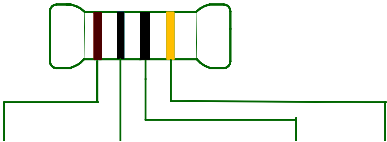
色环标识图
