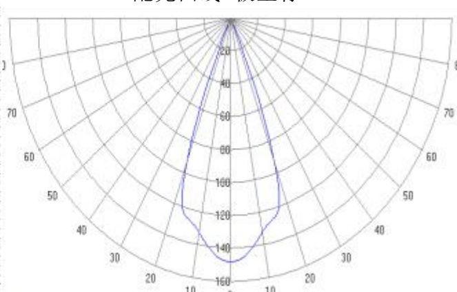
配光曲线-极坐标
