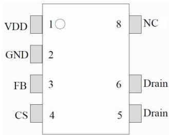
SOP-7 俯视图
