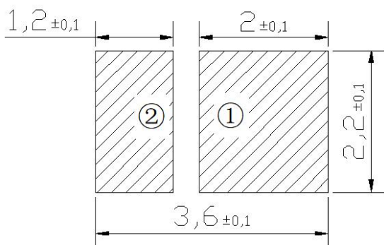
焊盘建议大小
