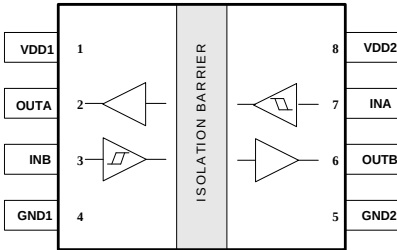
图 2. CMT8021NXL 管脚
