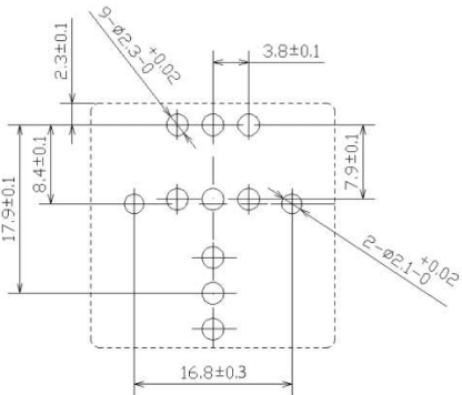
孔位图(光背 pcb 脚)
