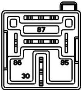
底视图(光背 pcb 脚)
