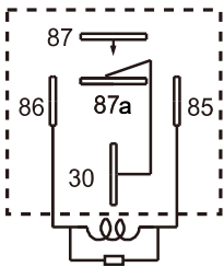
带电阻型
