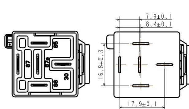
底视图(铁背长脚)
