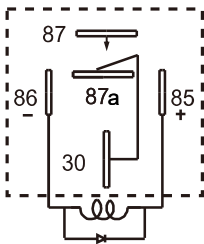
带二极管型 (D2)
