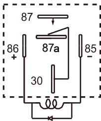
带二极管型 (D1)
