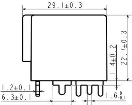
PCB脚外形图
