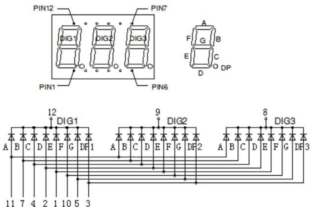
D3631A/B原理图
