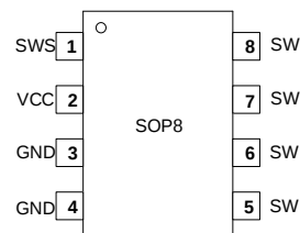
GP7596XB 管脚封装图
