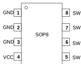
GP7596X 管脚封装图
