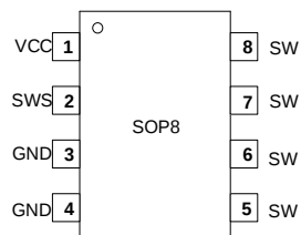
GP7596XA 管脚封装图
