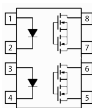
原理图
