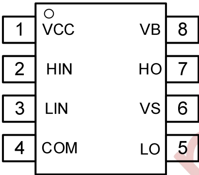
图 7-1 8-脚 SOP8 顶视图
