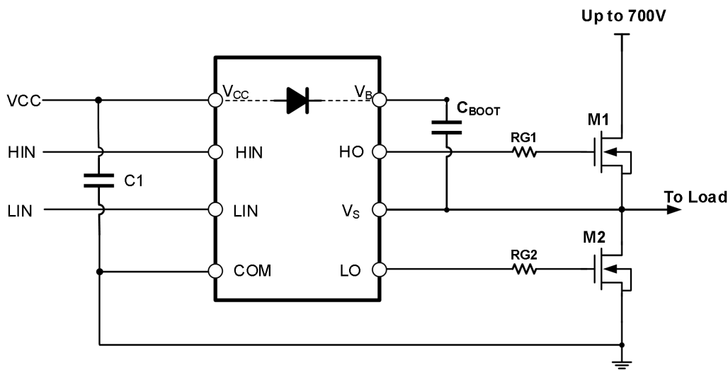
图 10-2 高速风筒专用电机驱动芯片 GG1000 典型应用电路图
