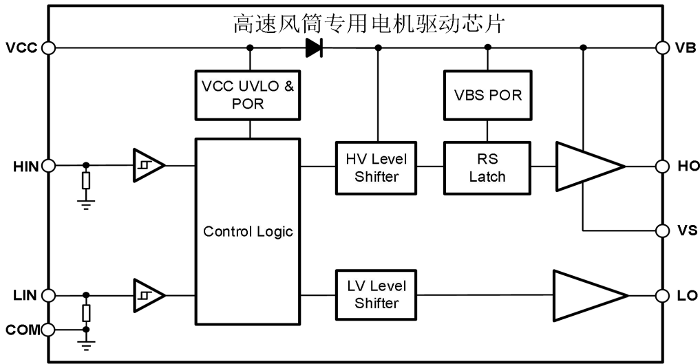
图 10-1 高速风筒专用电机驱动芯片 GG1000 的功能框图
