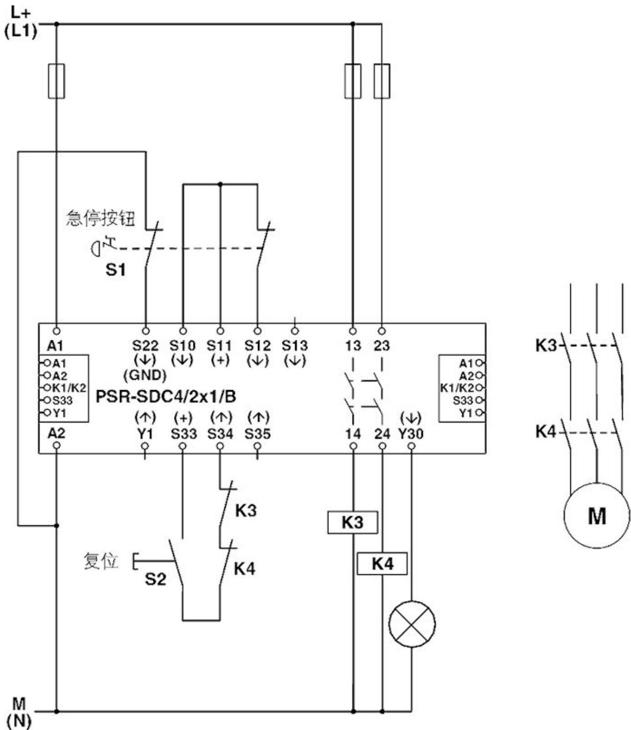
电路图
