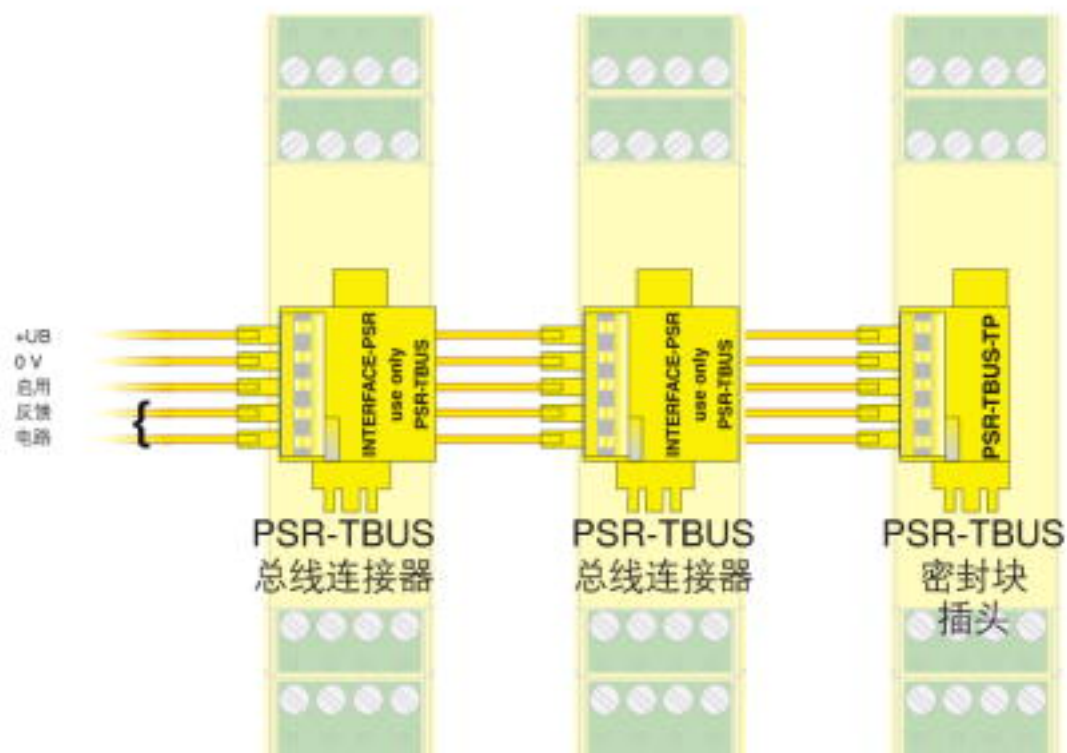
接线图
