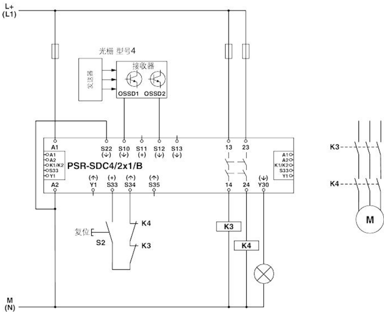
电路图
