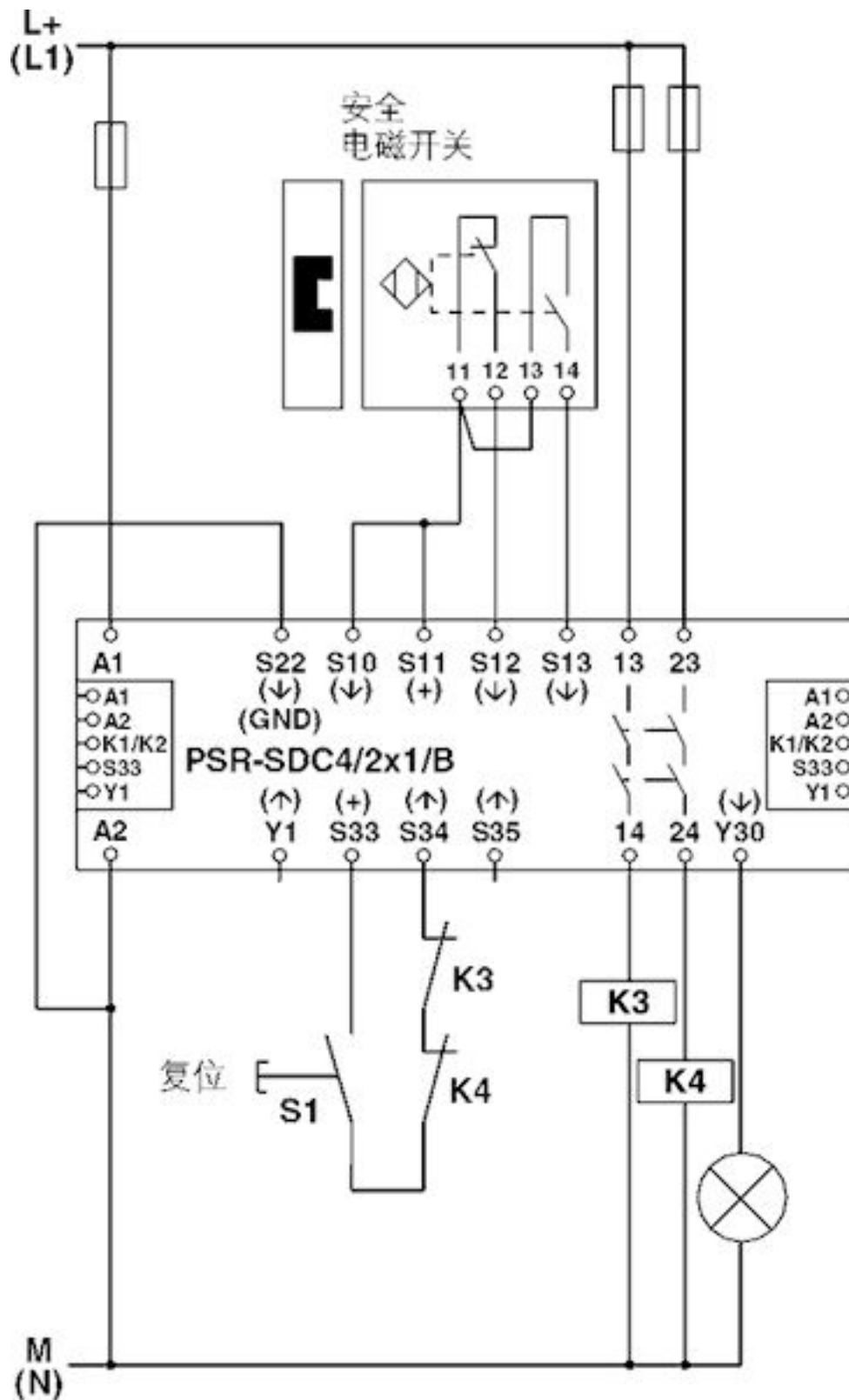
电路图
